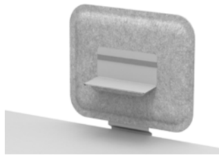
Option: Akustikbaffel mit Multibox-Halterung mit Multibox aus Formvlies und Gummiband
